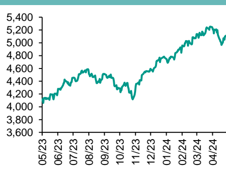
标普500走势图
